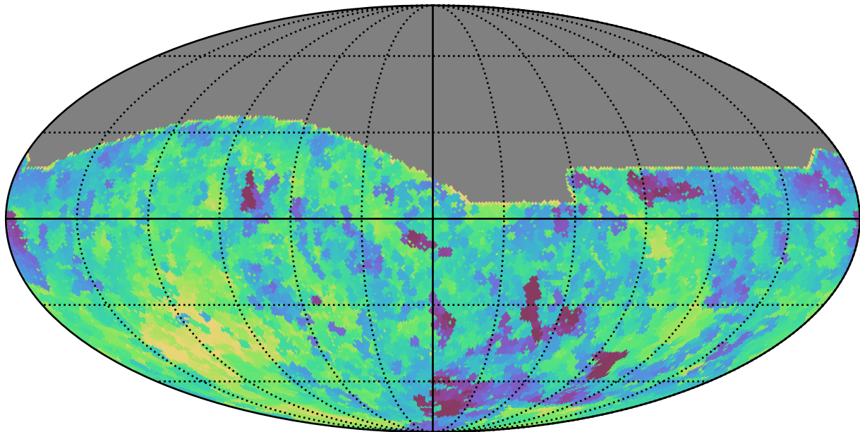
weather_cloudso0v3.4_10yrs All sky i band: Min saturation_mag
