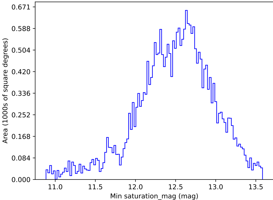
weather_cloudso0v3.4_10yrs All sky i band: Min saturation_mag
