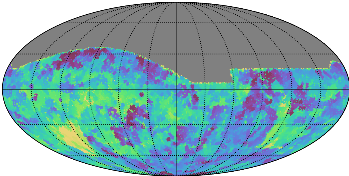
weather_cloudso0v3.4_10yrs All sky g band: Min saturation_mag
