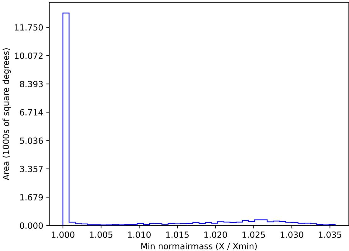
weather_cloudso0v3.4_10yrs WFD z band: Min normairmass
