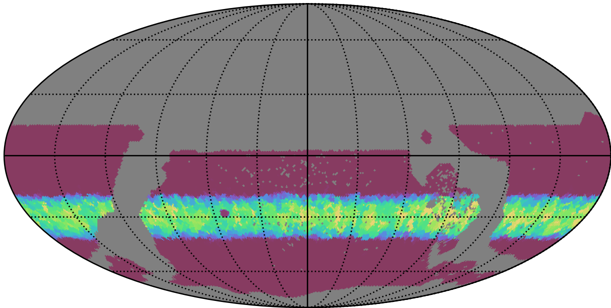
weather_cloudso0v3.4_10yrs WFD y band: Min normairmass
