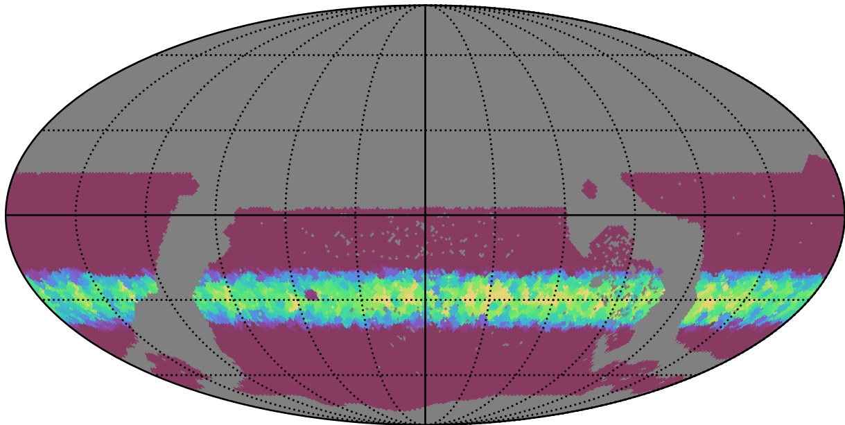
weather_cloudso0v3.4_10yrs WFD r band: Min normairmass
