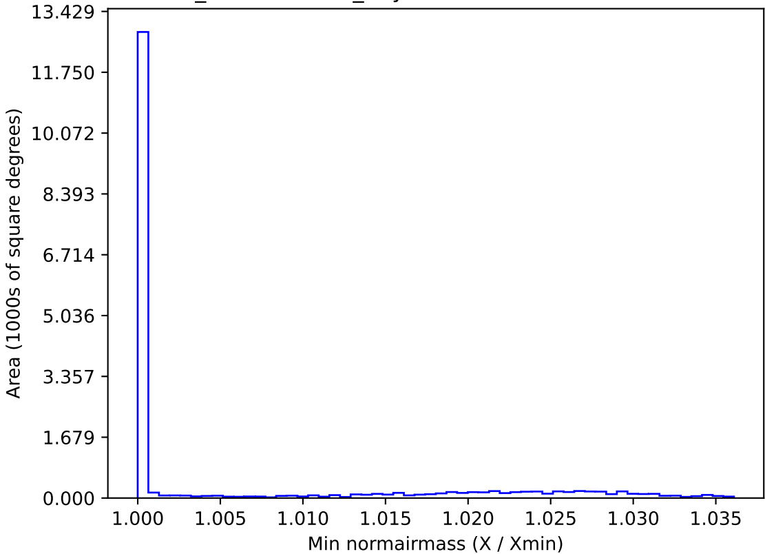
weather_cloudso0v3.4_10yrs WFD r band: Min normairmass
