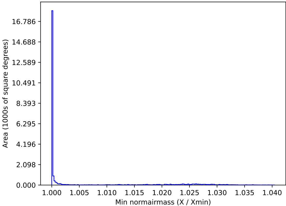
weather_cloudso0v3.4_10yrs All sky z band: Min normairmass
