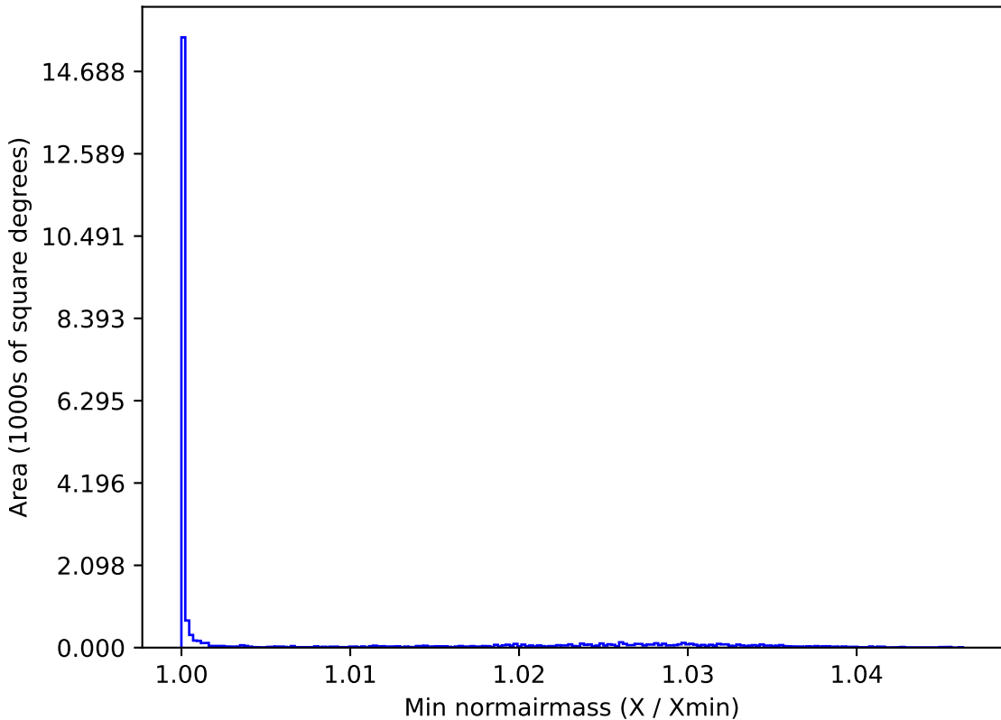
weather_cloudso0v3.4_10yrs All sky y band: Min normairmass
