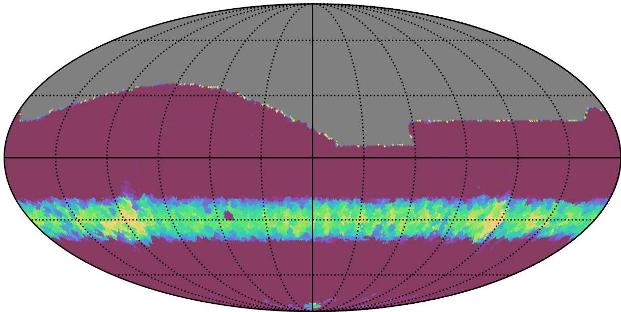
weather_cloudso0v3.4_10yrs All sky i band: Min normairmass
