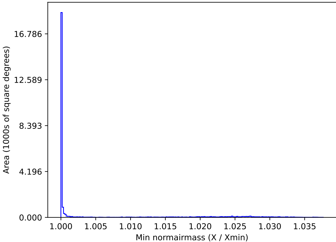
weather_cloudso0v3.4_10yrs All sky i band: Min normairmass
