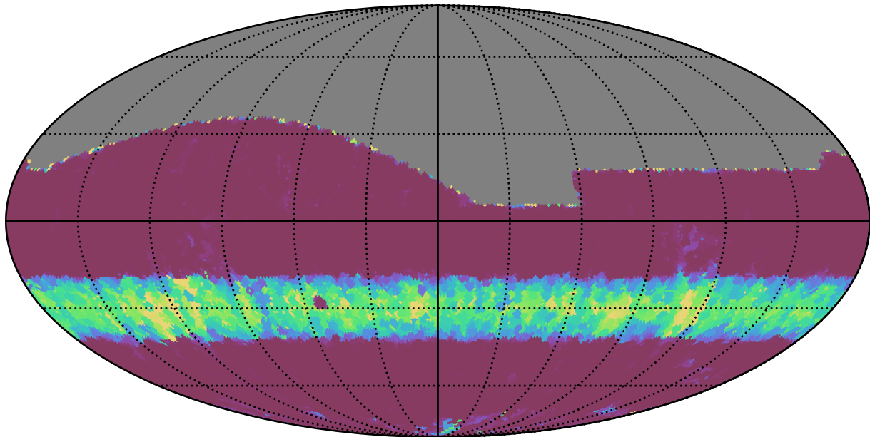
weather_cloudso0v3.4_10yrs All sky g band: Min normairmass
