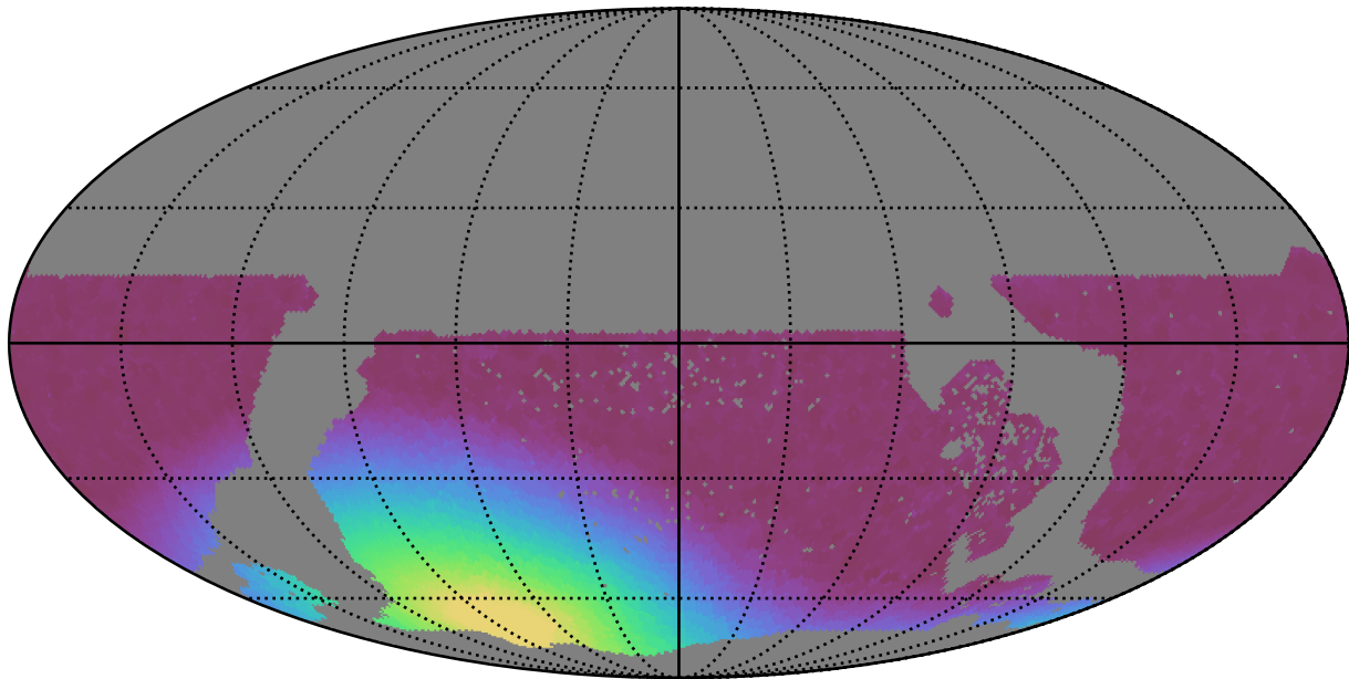
weather_cloudso0v3.4_10yrs WFD y band: Min moonDistance
