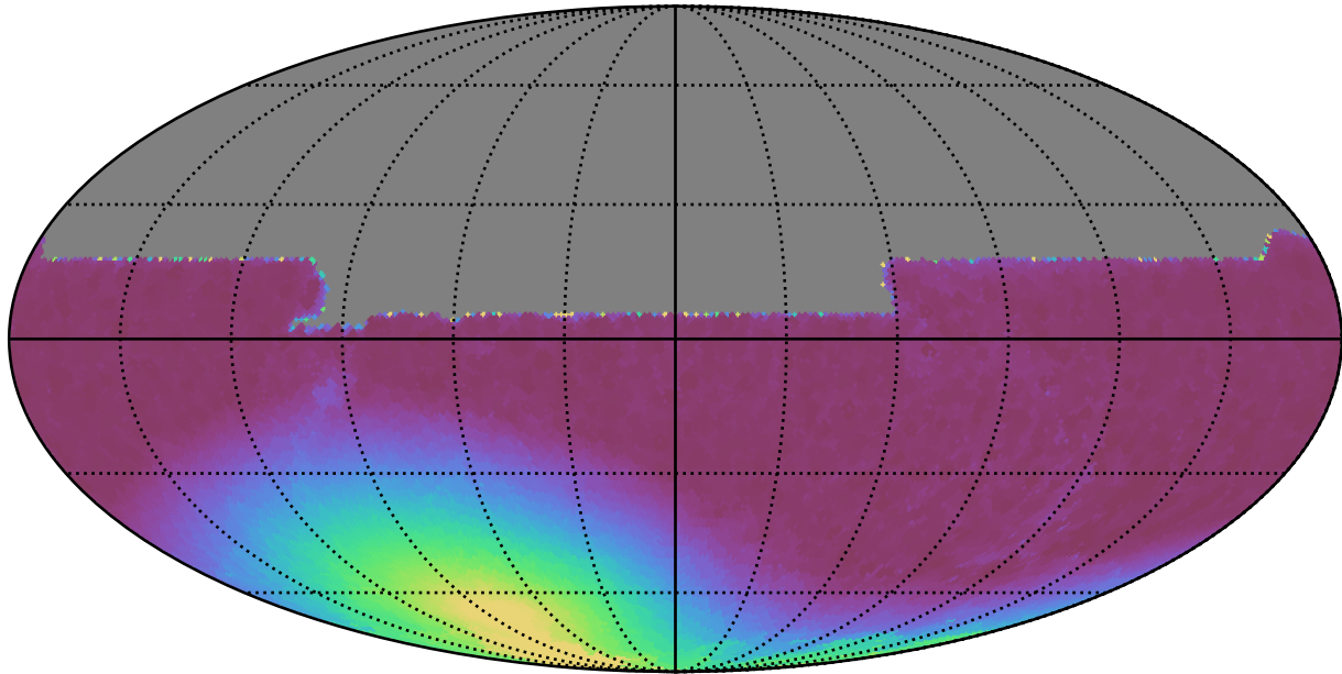
weather_cloudso0v3.4_10yrs All sky y band: Min moonDistance
