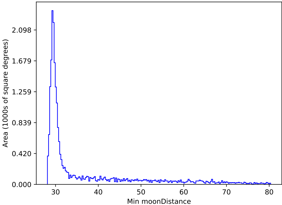
weather_cloudso0v3.4_10yrs All sky y band: Min moonDistance
