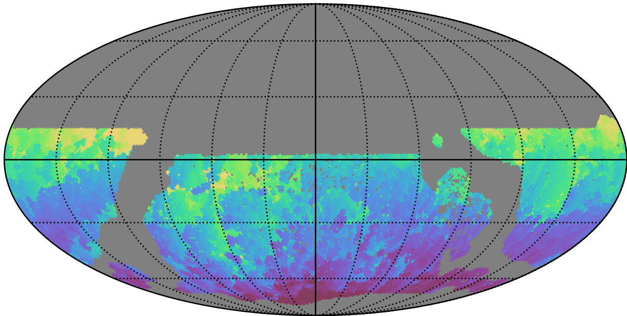
weather_cloudso0v3.4_10yrs WFD z band: Min HA
