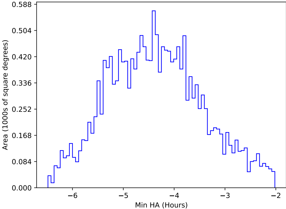
weather_cloudso0v3.4_10yrs WFD z band: Min HA
