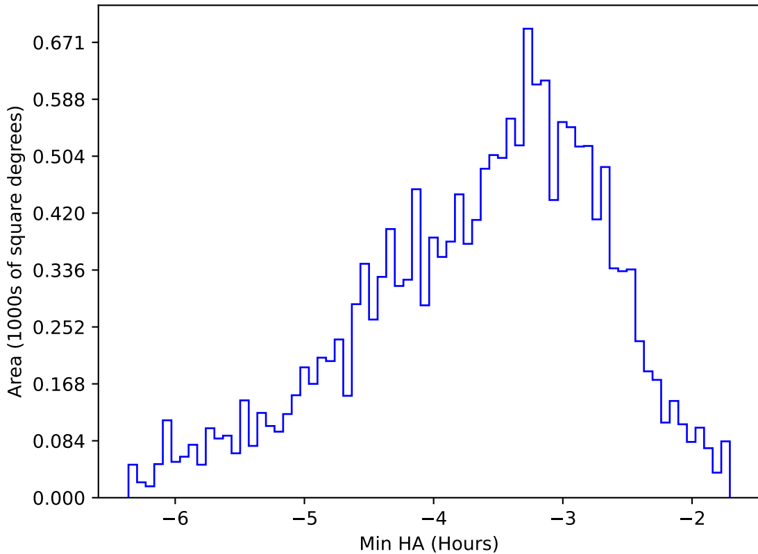
weather_cloudso0v3.4_10yrs WFD y band: Min HA
