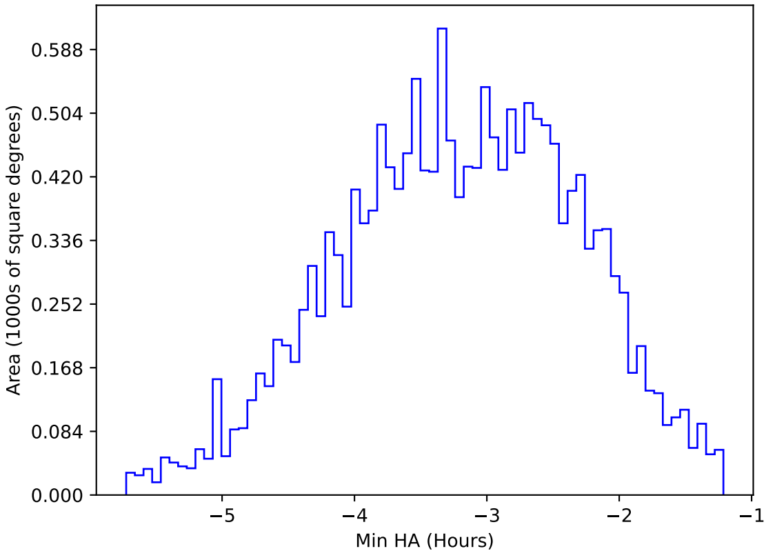
weather_cloudso0v3.4_10yrs WFD u band: Min HA
