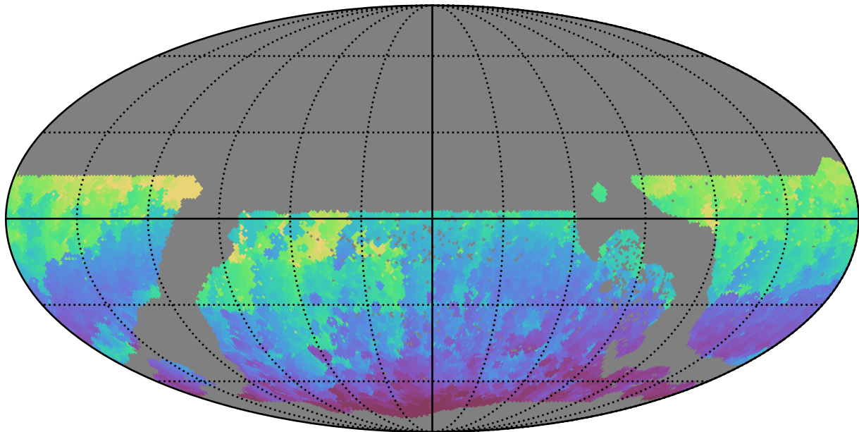
weather_cloudso0v3.4_10yrs WFD i band: Min HA
