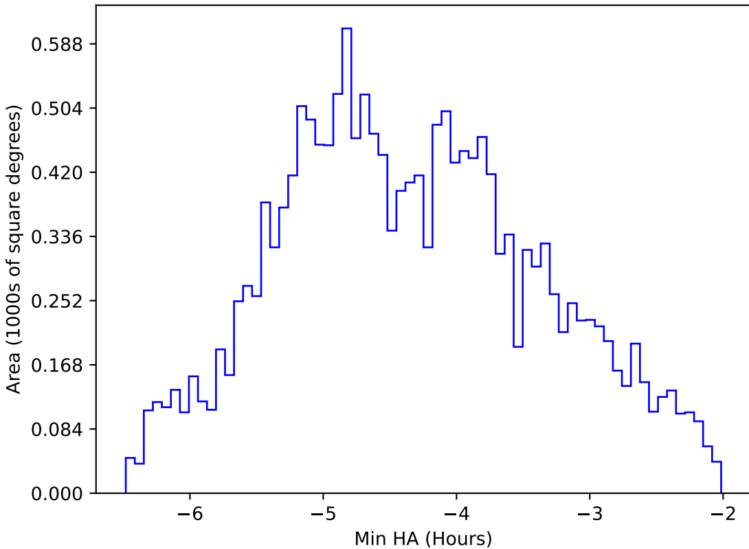
weather_cloudso0v3.4_10yrs WFD i band: Min HA
