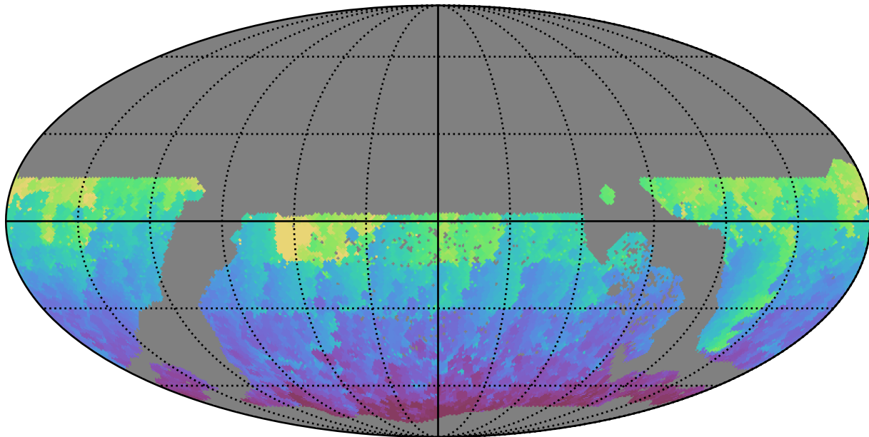
weather_cloudso0v3.4_10yrs WFD g band: Min HA
