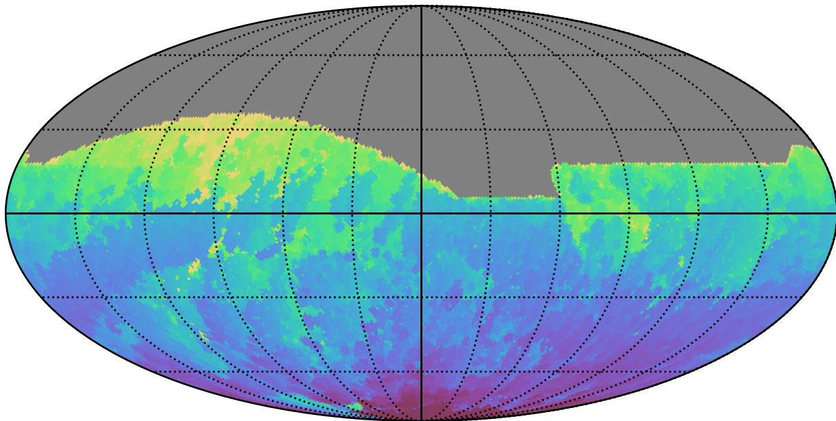
weather_cloudso0v3.4_10yrs All sky z band: Min HA
