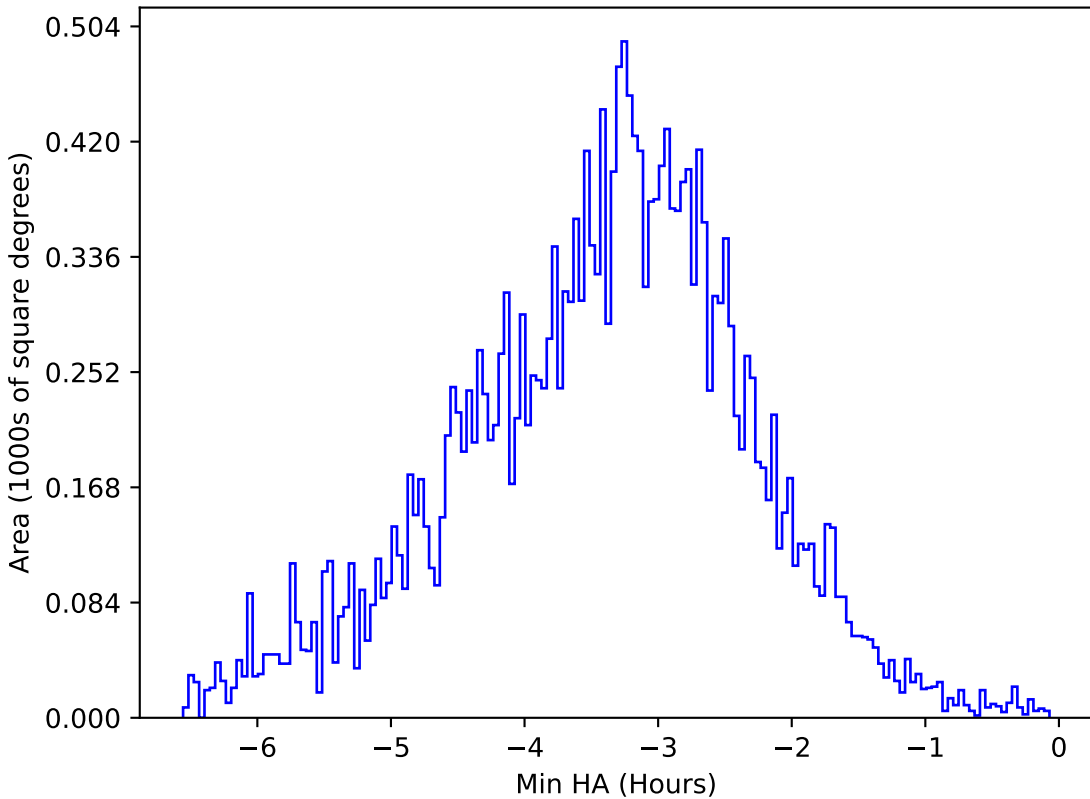
weather_cloudso0v3.4_10yrs All sky y band: Min HA
