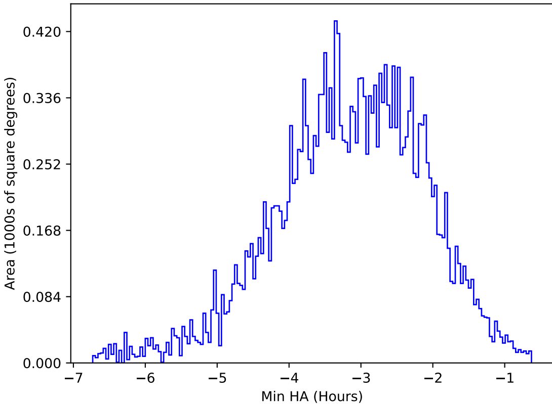
weather_cloudso0v3.4_10yrs All sky u band: Min HA
