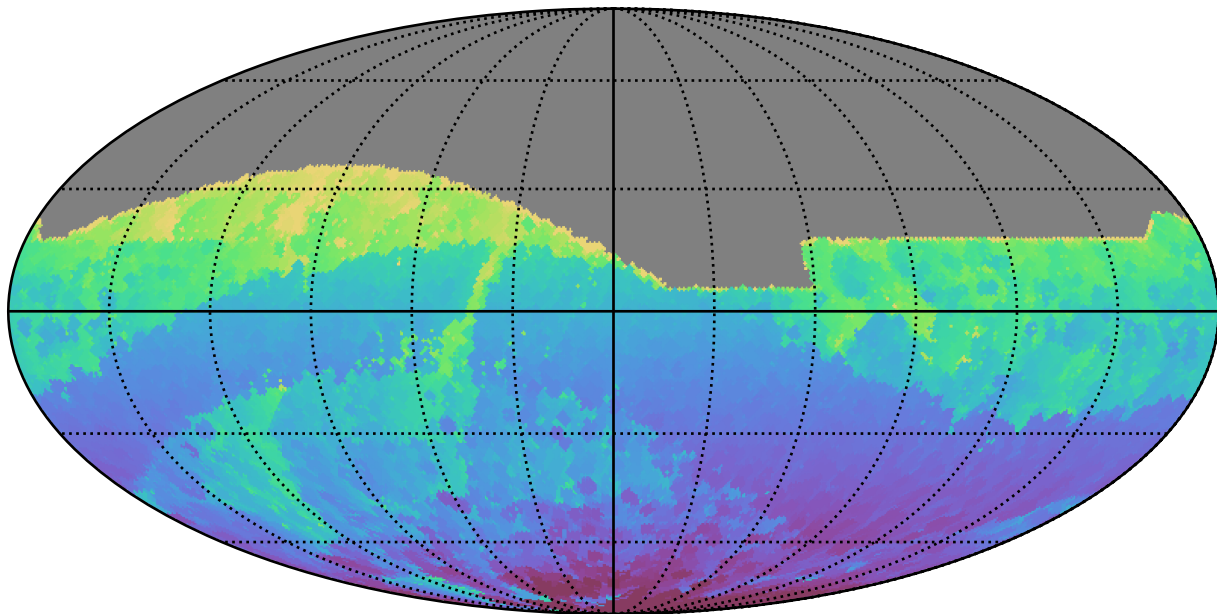
weather_cloudso0v3.4_10yrs All sky r band: Min HA
