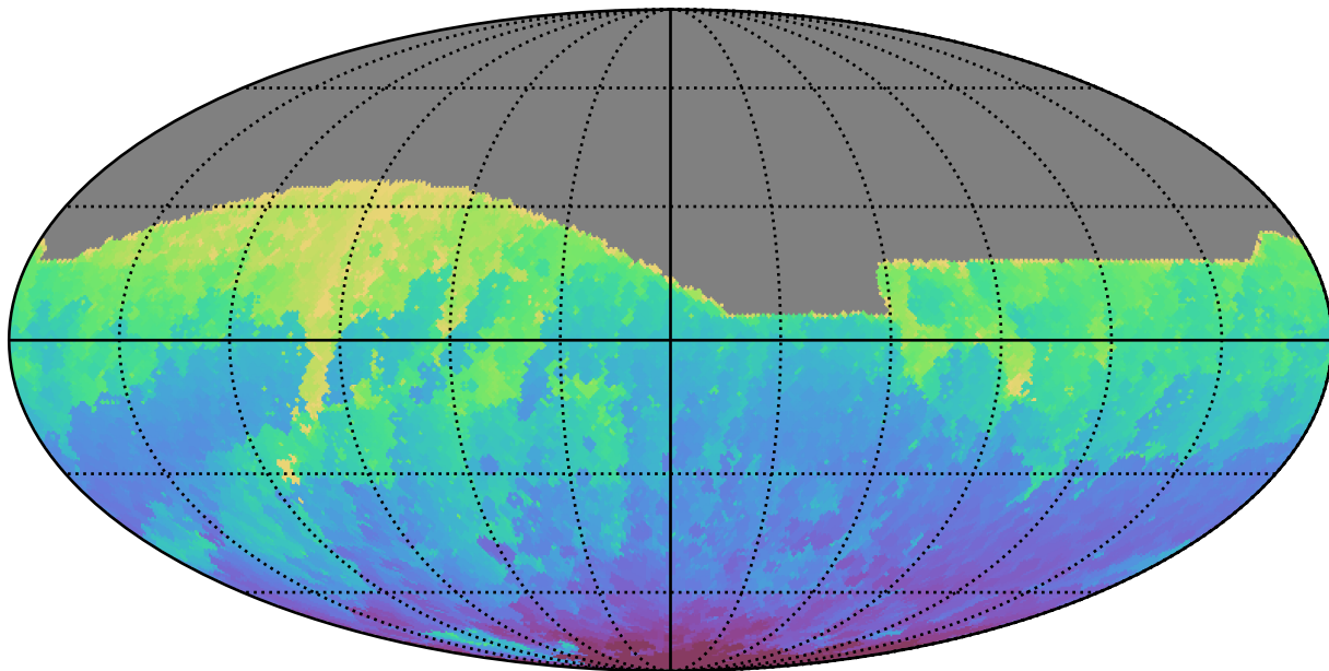
weather_cloudso0v3.4_10yrs All sky i band: Min HA
