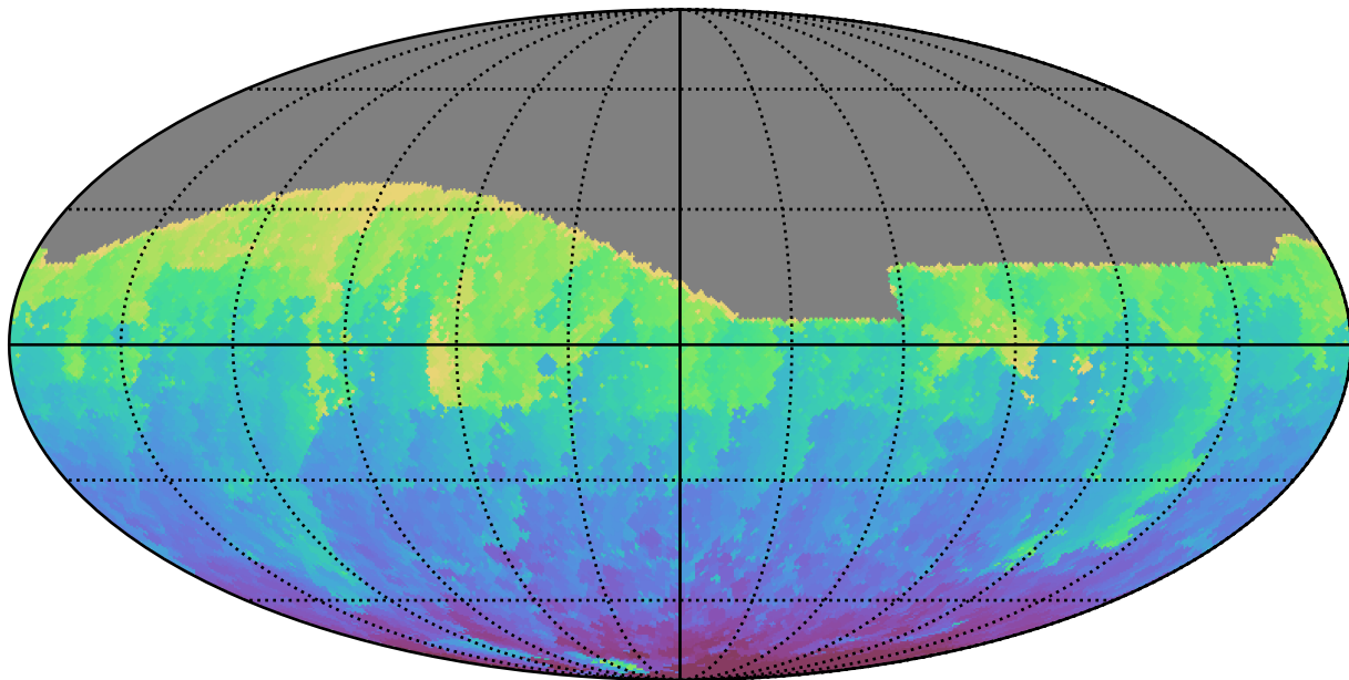
weather_cloudso0v3.4_10yrs All sky g band: Min HA
