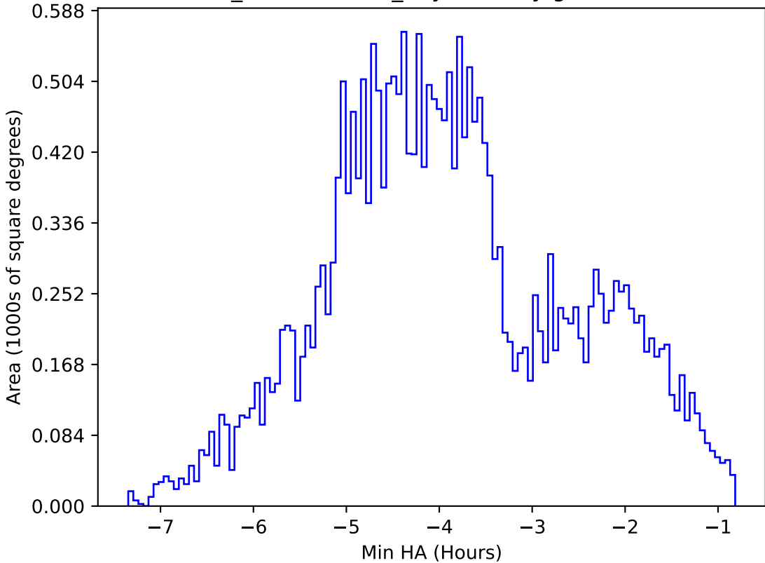
weather_cloudso0v3.4_10yrs All sky g band: Min HA
