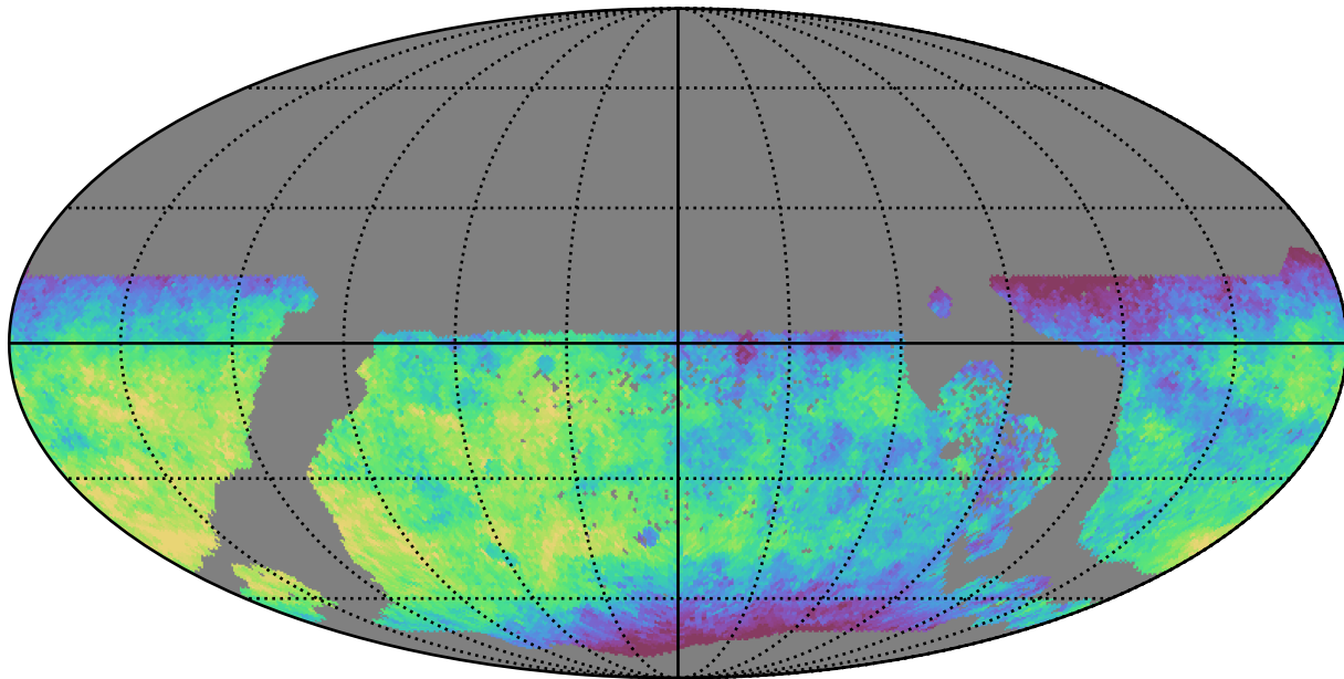
weather_cloudso0v3.4_10yrs WFD y band: Median saturation_mag
