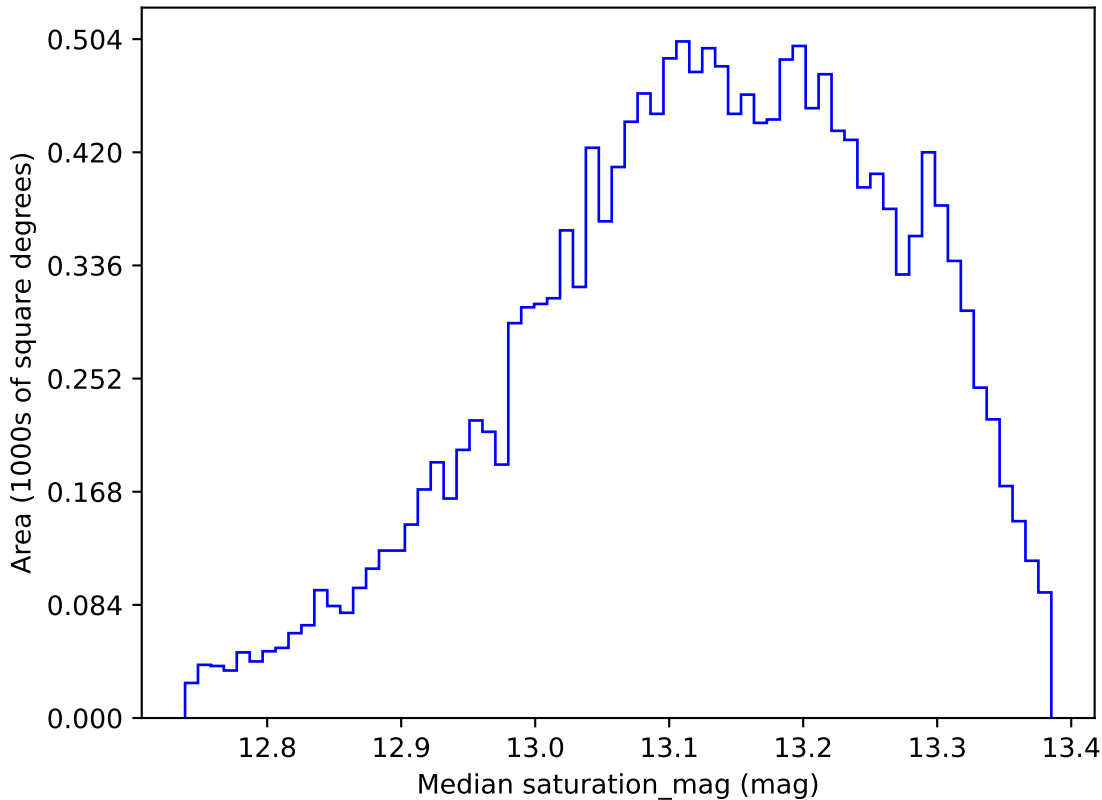
weather_cloudso0v3.4_10yrs WFD y band: Median saturation_mag
