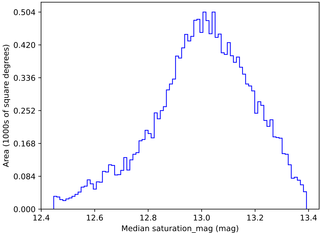
weather_cloudso0v3.4_10yrs WFD u band: Median saturation_mag
