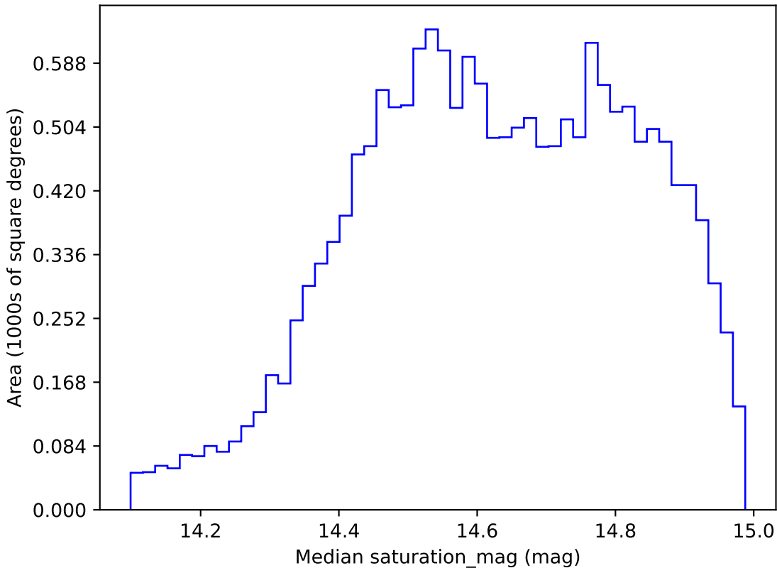
weather_cloudso0v3.4_10yrs WFD r band: Median saturation_mag
