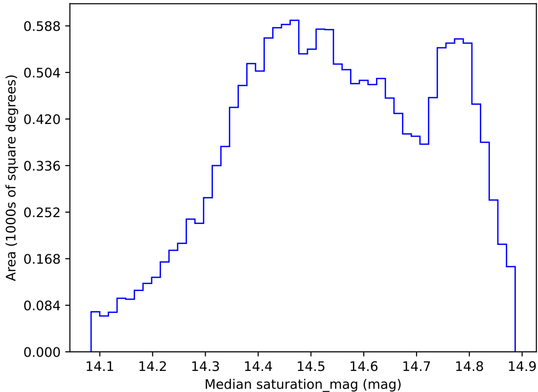
weather_cloudso0v3.4_10yrs WFD i band: Median saturation_mag
