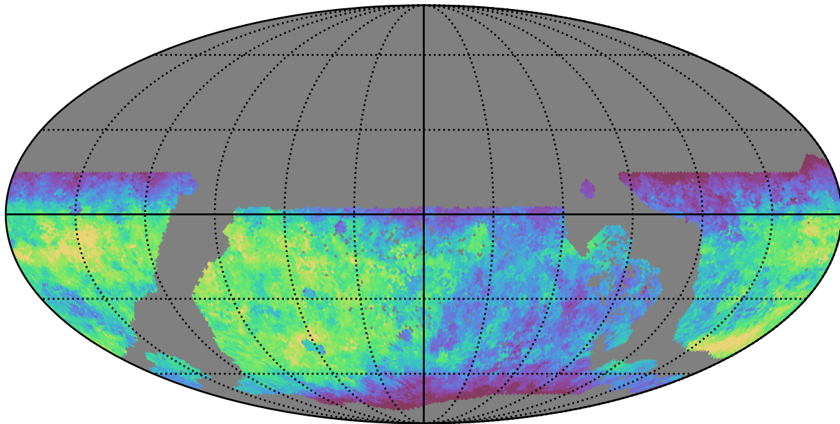
weather_cloudso0v3.4_10yrs WFD g band: Median saturation_mag
