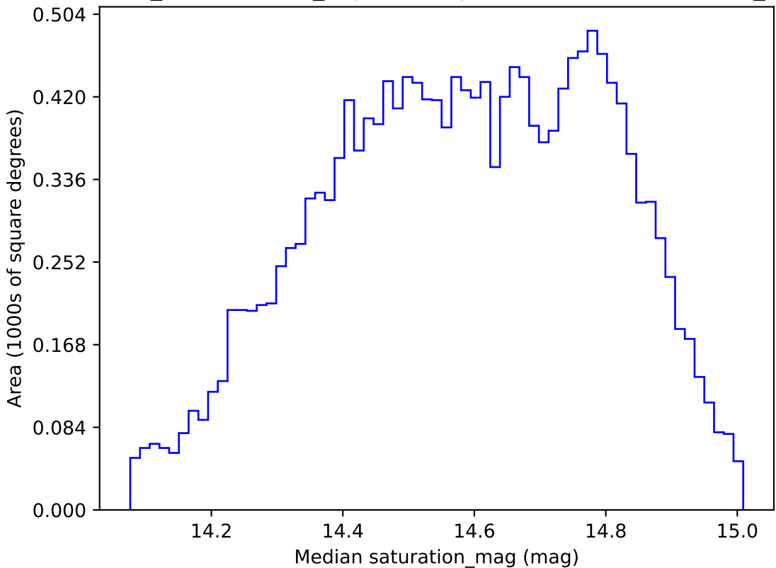
weather_cloudso0v3.4_10yrs WFD g band: Median saturation_mag
