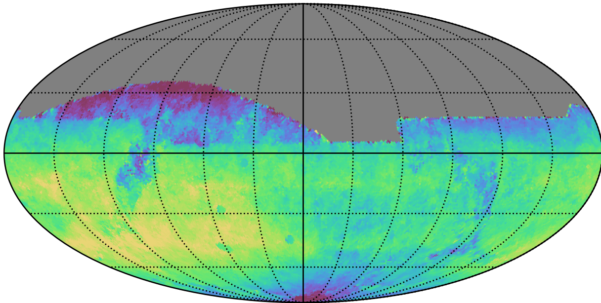
weather_cloudso0v3.4_10yrs All sky z band: Median saturation_mag
