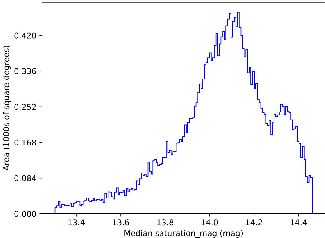
weather_cloudso0v3.4_10yrs All sky z band: Median saturation_mag
