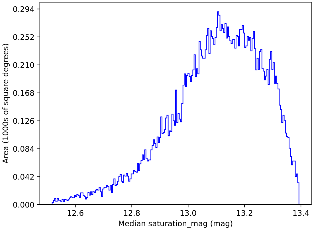
weather_cloudso0v3.4_10yrs All sky y band: Median saturation_mag
