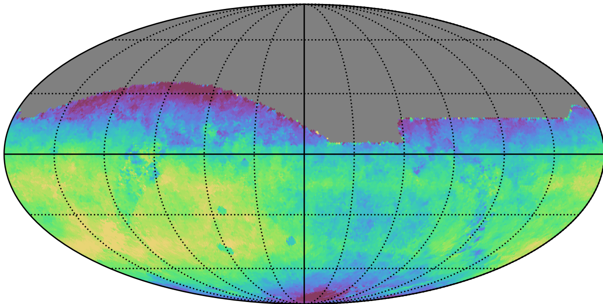
weather_cloudso0v3.4_10yrs All sky i band: Median saturation_mag
