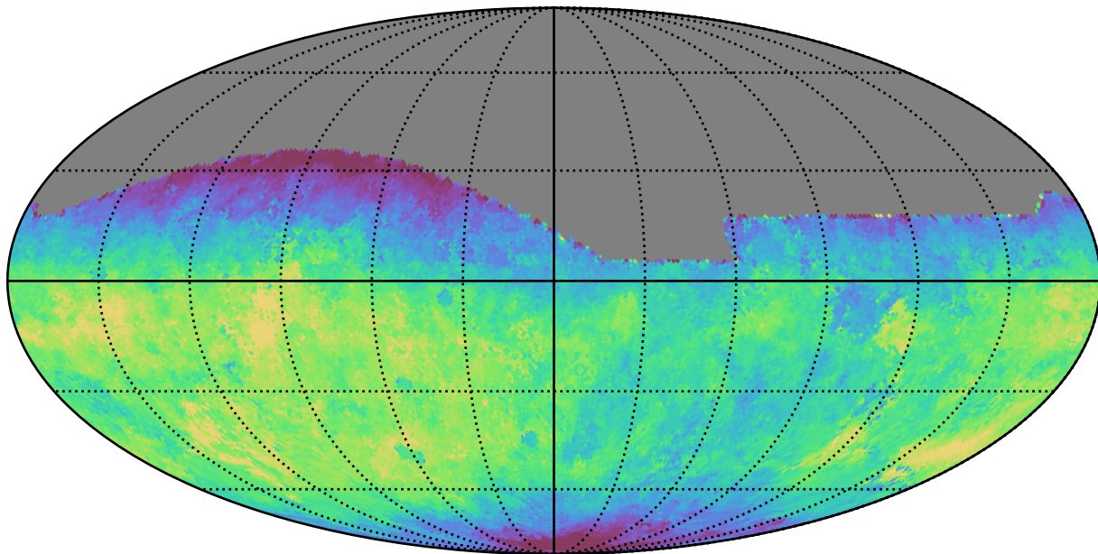
weather_cloudso0v3.4_10yrs All sky g band: Median saturation_mag
