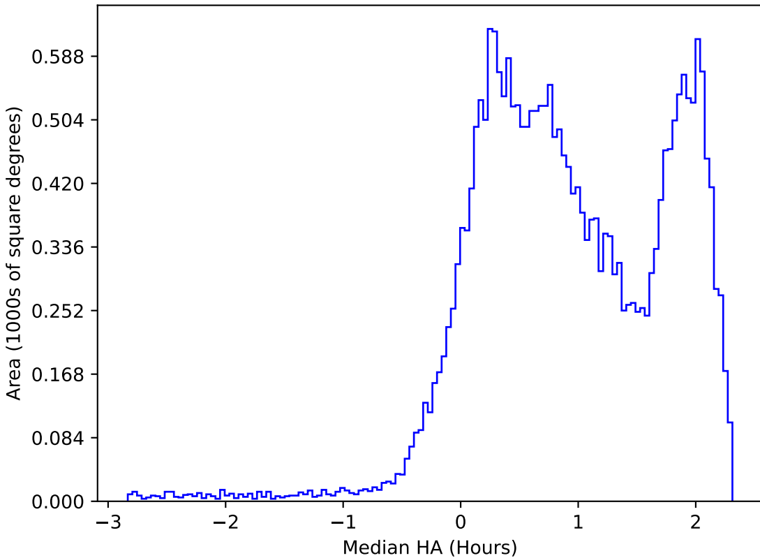
weather_cloudso0v3.4_10yrs All sky i band: Median HA
