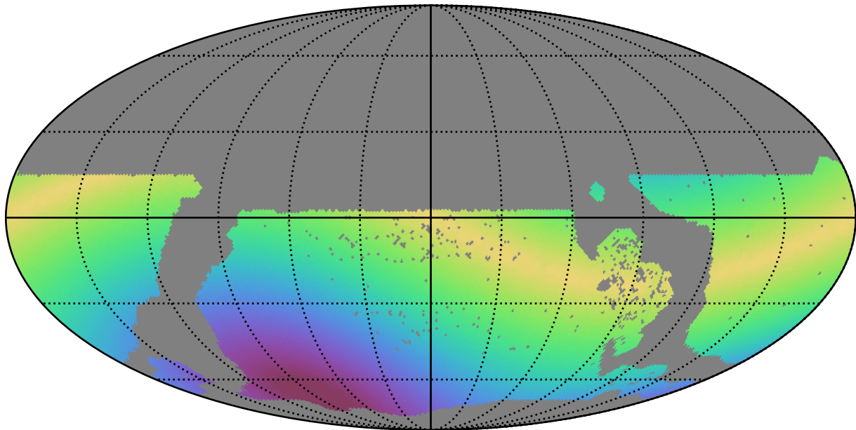
weather_cloudso0v3.4_10yrs WFD z band: Max solarElong
