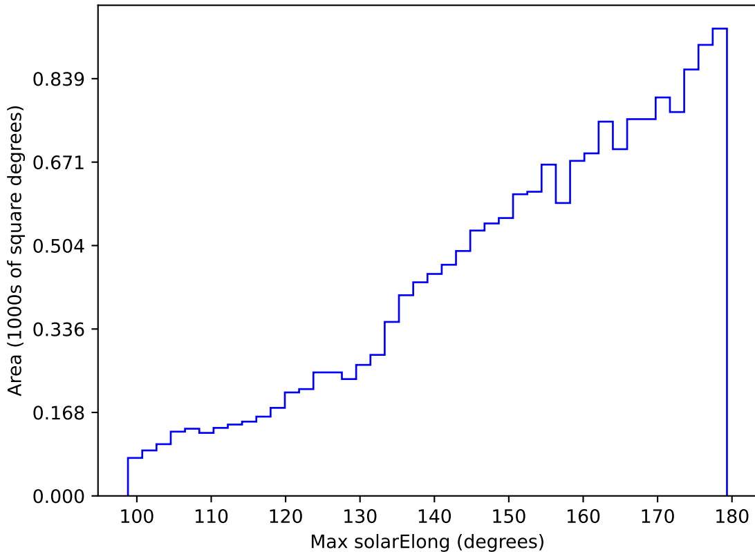
weather_cloudso0v3.4_10yrs WFD y band: Max solarElong
