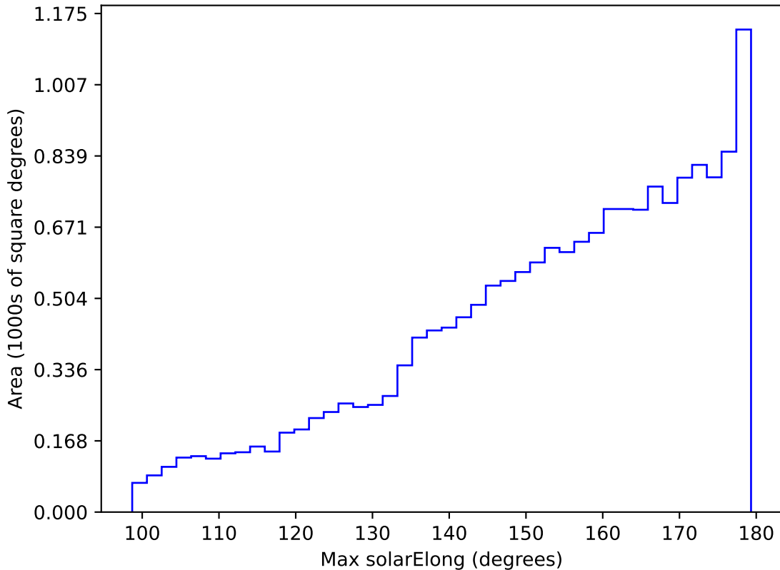
weather_cloudso0v3.4_10yrs WFD i band: Max solarElong
