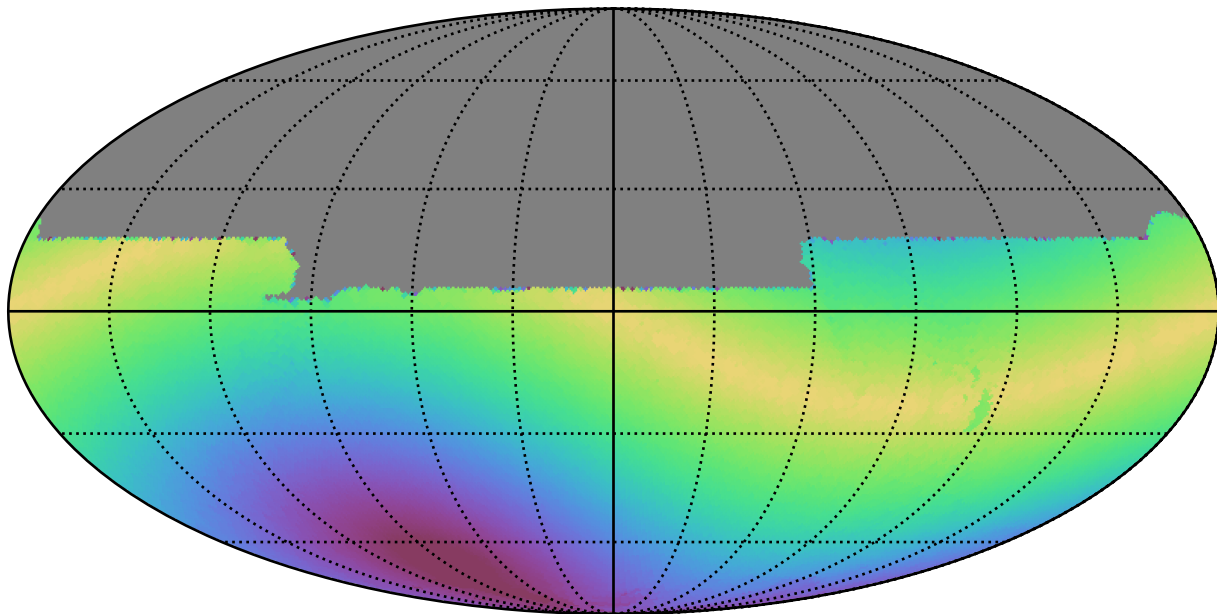
weather_cloudso0v3.4_10yrs All sky y band: Max solarElong
