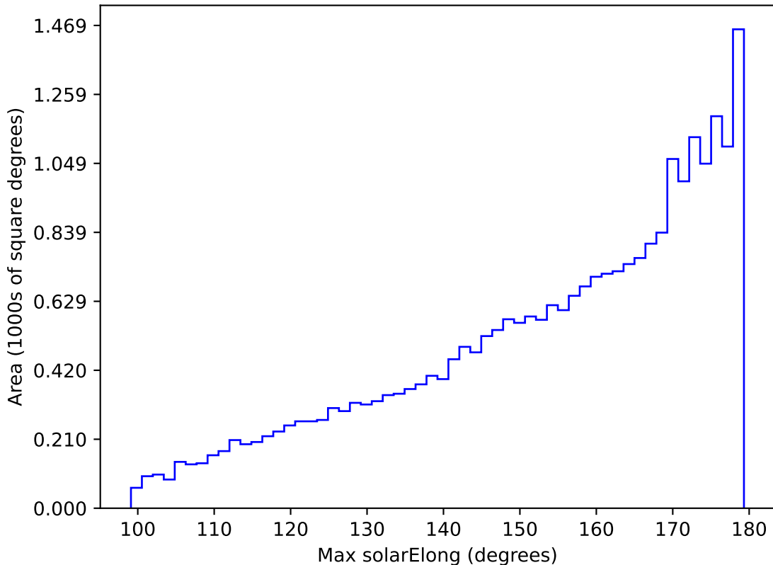
weather_cloudso0v3.4_10yrs All sky i band: Max solarElong
