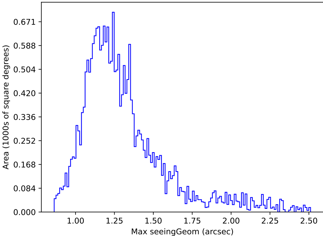
weather_cloudso0v3.4_10yrs Yr 1 y band: Max seeingGeom
