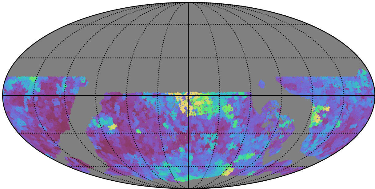
weather_cloudso0v3.4_10yrs WFD y band: Max seeingEff
