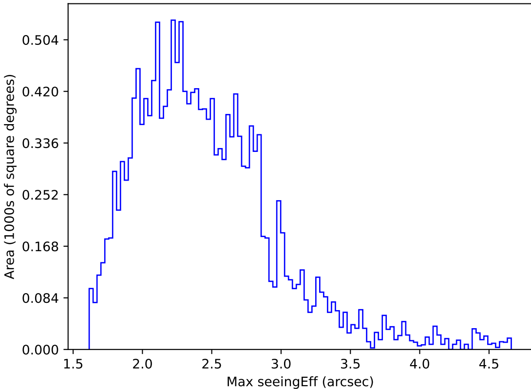
weather_cloudso0v3.4_10yrs WFD y band: Max seeingEff
